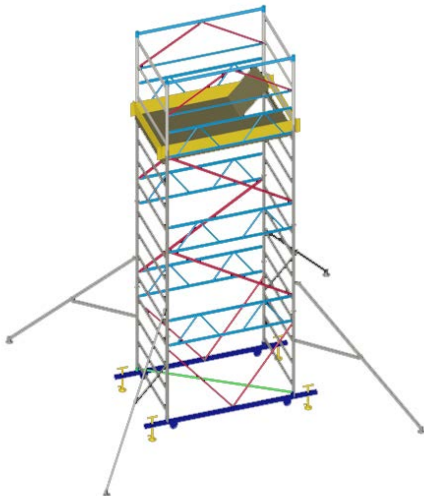
Figura 4.2-8 Rappresentazione del trabattello completo (esempio con 3 impalcati)
