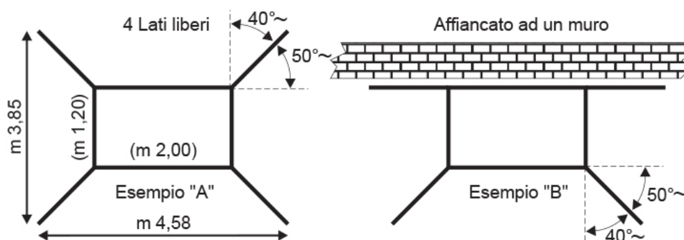
Figura 4.2-6 Disposizione delle staffe stabilizzatrici
