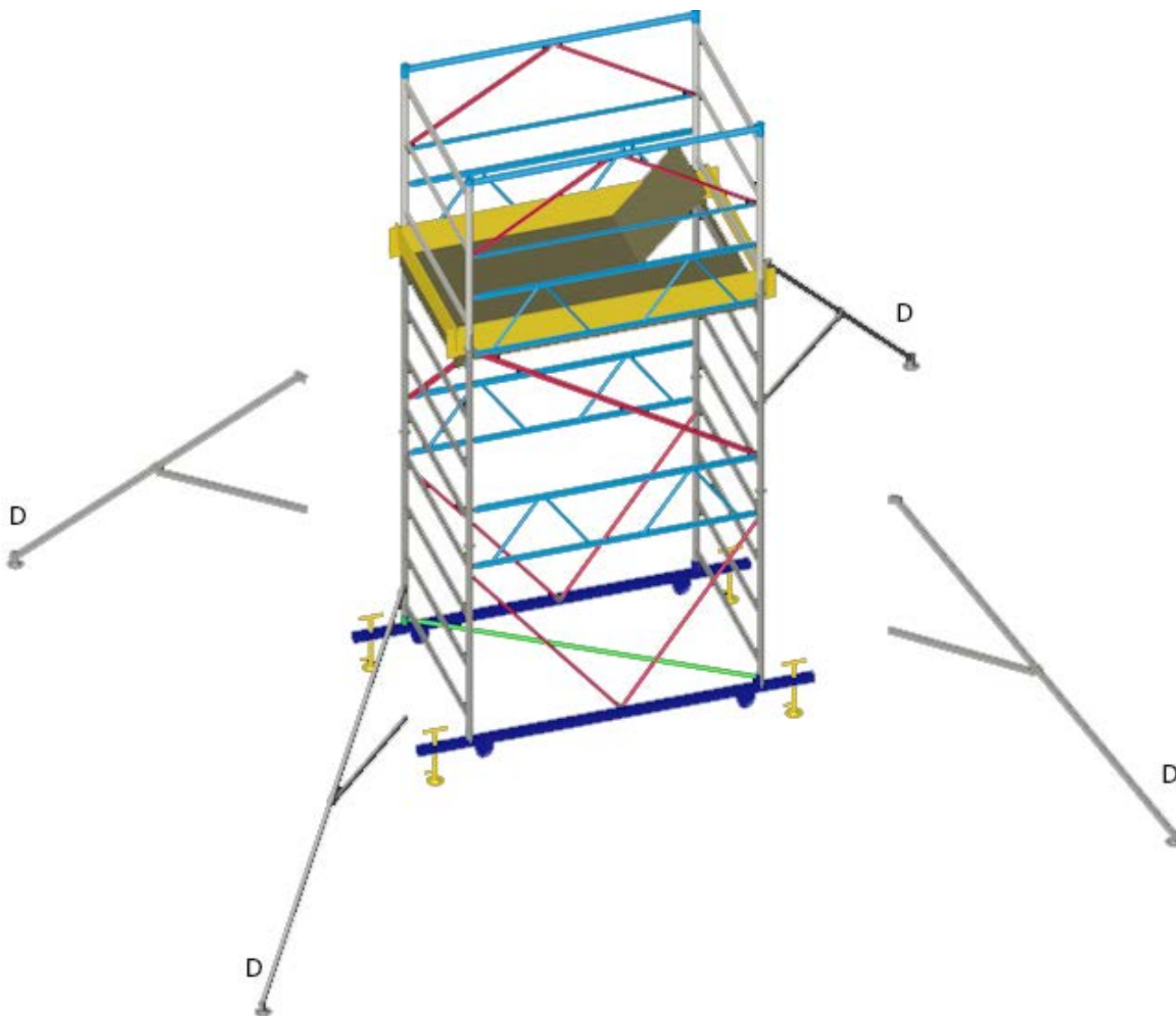
Figura 4.2-6 Fase di montaggio degli stabilizzatori
