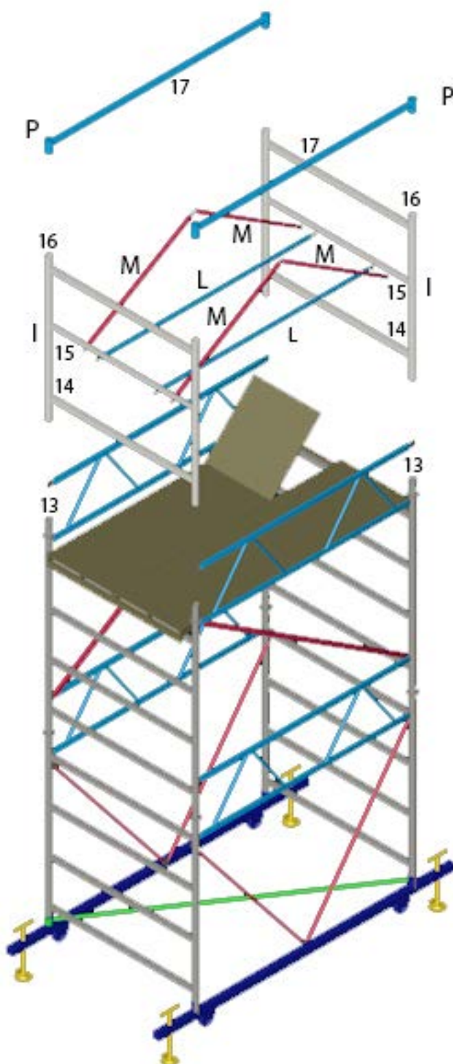
Figura 4.2-4 Fase di montaggio dei parapetti
