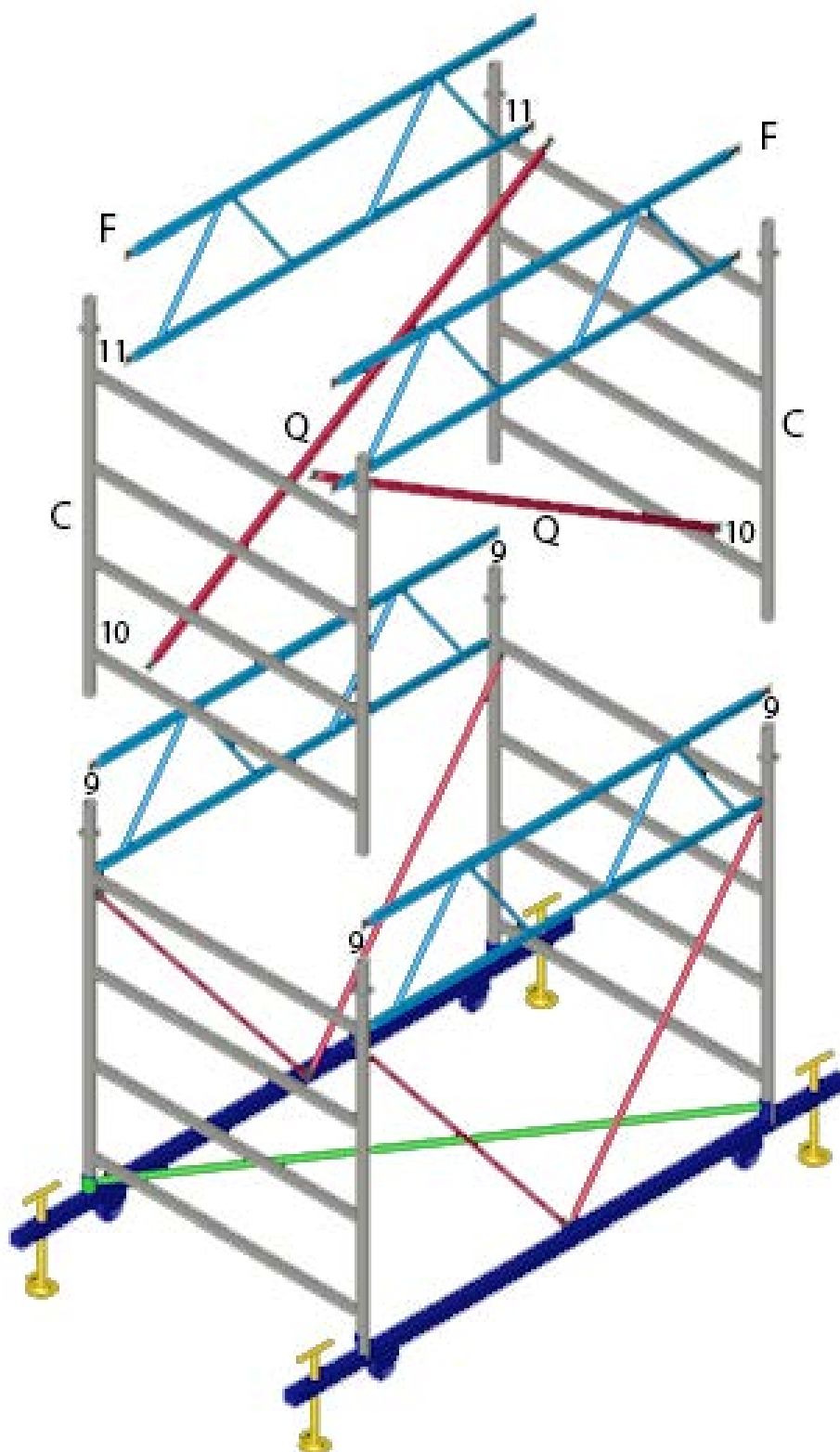
Figura 4.2-2 Fase di montaggio del secondo livello
