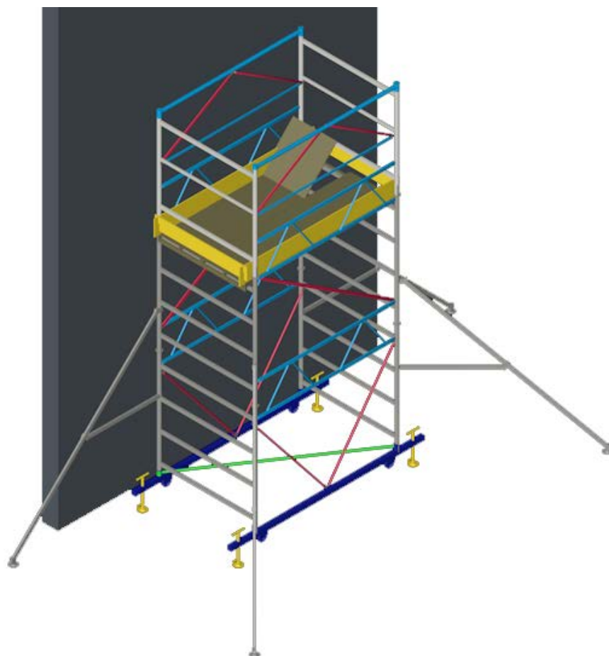
Figura 4.2-9 Rappresentazione del trabattello completo (posizionamento in aderenza)
