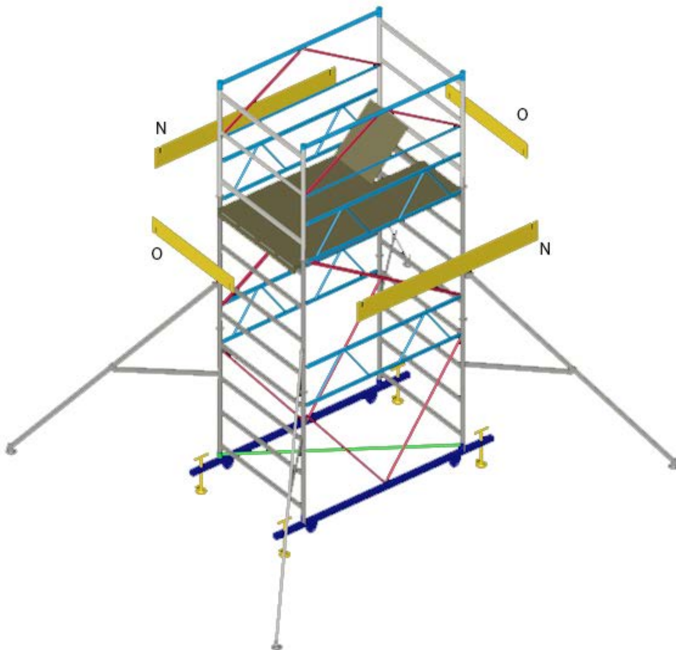
Figura 4.2-5 Fase di montaggio dei fermapiedi
