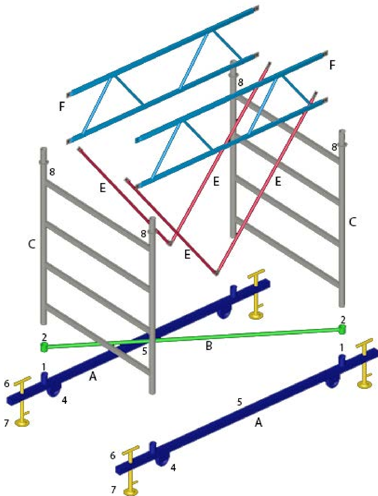
Figura 4.2-1 Fase di montaggio dell'elemento di base e del primo livello
