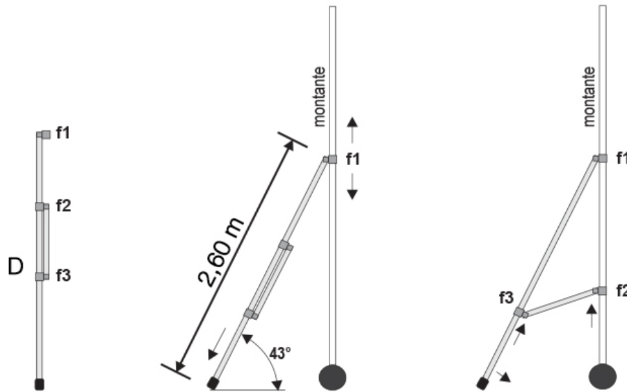
Figura 4.2-5 Montaggio delle staffe stabilizzatrici
