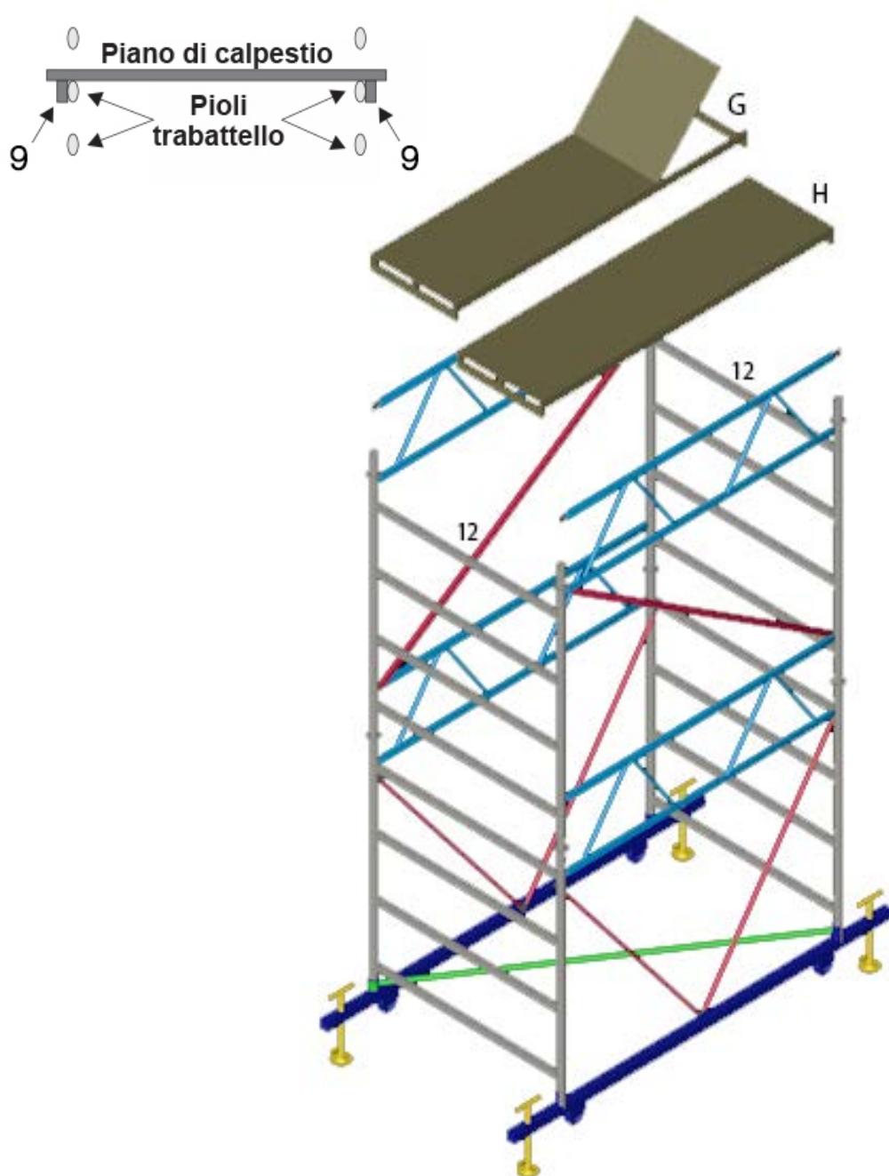
Figura 4.2-3 Fase di montaggio del piano di lavoro
